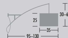
Wall lamp EMIWVL61125 1 x E27
