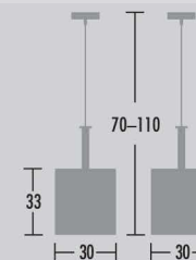
Pendant lamp EMIPL61113 1 x E27
